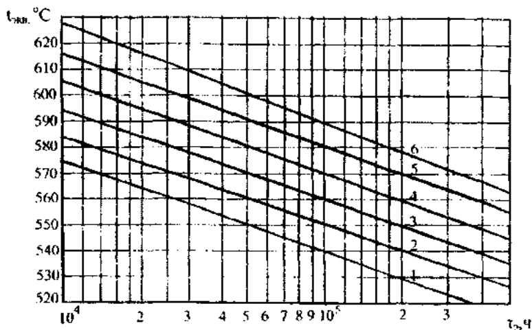
Рисунок 8.2 - Номограмма для определения эквивалентной температуры эксплуатации металла труб из стали 12Х1МФ по структуре и доли молибдена в карбидах.
