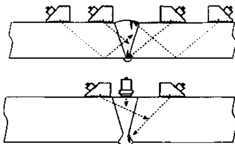
Рисунок 4.29 - Схемы контроля
