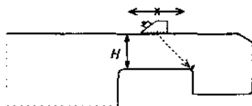
Рисунок 4.20 - Схема контроля
