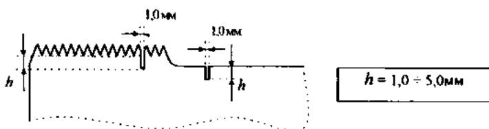
Рисунок 4.19 - Схема образца
