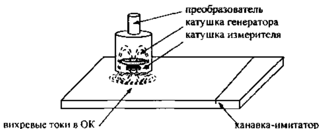
Рисунок 4.63 - Настройка «компенсации» и чувствительности
