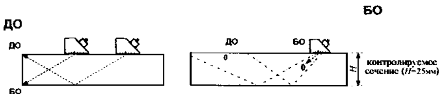
БО -ближний отражатель, ДО -дальний отражатель
