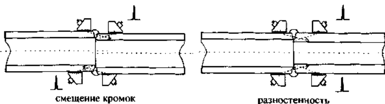
Рисунок 4.34 - Контроль смещения кромок и разностенности
