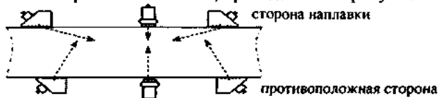
Рисунок 4.36 - Схема контроля
