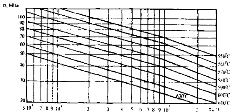
Рисунок 8.8. График для определения времени до разрушения металла труб из стали 12X18H12T в исходном состоянии
