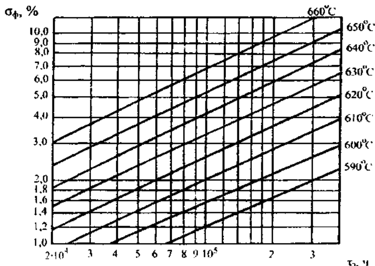
Рисунок 8.5 - Номограмма для определения эквивалентной температуры эксплуатации металла труб из стали 12X18Н12Т по количеству \sigma_{\phi}
