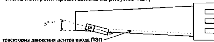
Рисунок 4.27 - Схема контроля
