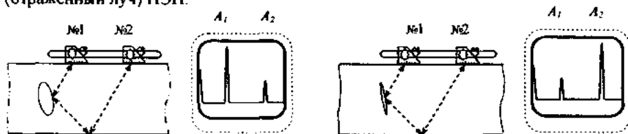
Рисунок 4.12 - Определение коэффициента формы отражателя
