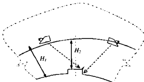
Рисунок 4.24 - Схема контроля
