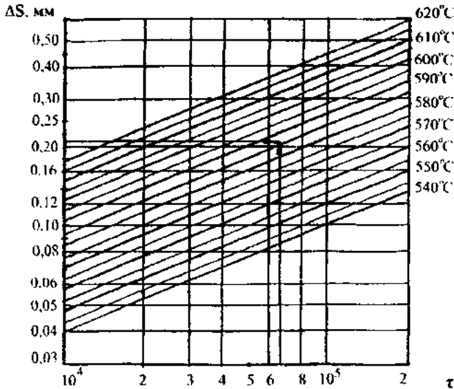
Рисунок 8.3. - График для определения эквивалентной температуры эксплуатации металла труб из стали 12Х1МФ по глубине коррозии
