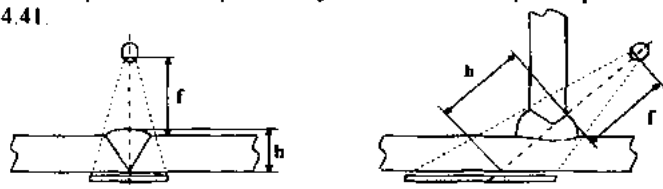
Рисунок 4.41 - Схемы контроля сварных швов металлоконструкций
