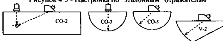
Рисунок 4.5 - Настройка по "эталонным" отражателям
